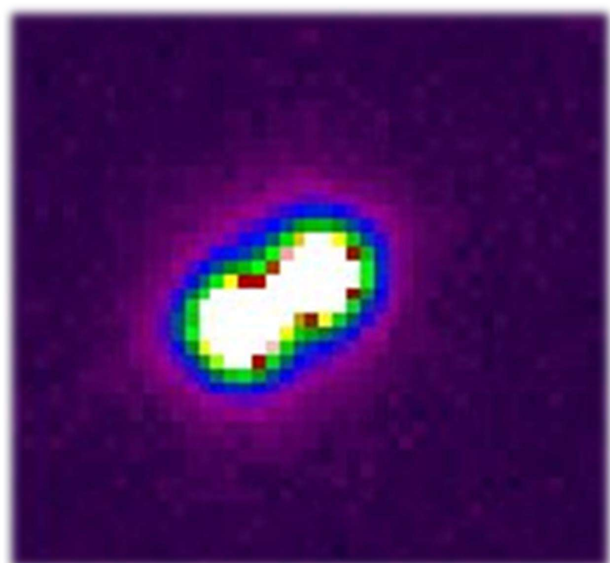
Fig. 3. Meer dan 67% van de sterren uit de nabije zonsomgeving behoren tot dubbele of meervoudige stersystemen. De zon heeft geen begeleider, wat haar vanuit dit standpunt uitzonderlijk maakt. Plus de 67% des étoiles de l'environnement solaire appartiennent à des systèmes d'étoiles doubles et multiples. Le Soleil n'a pas d'étoile-compagnon, ce qui la rend exceptionnelle vue sous cet angle. © NASA/JPL-Caltech
