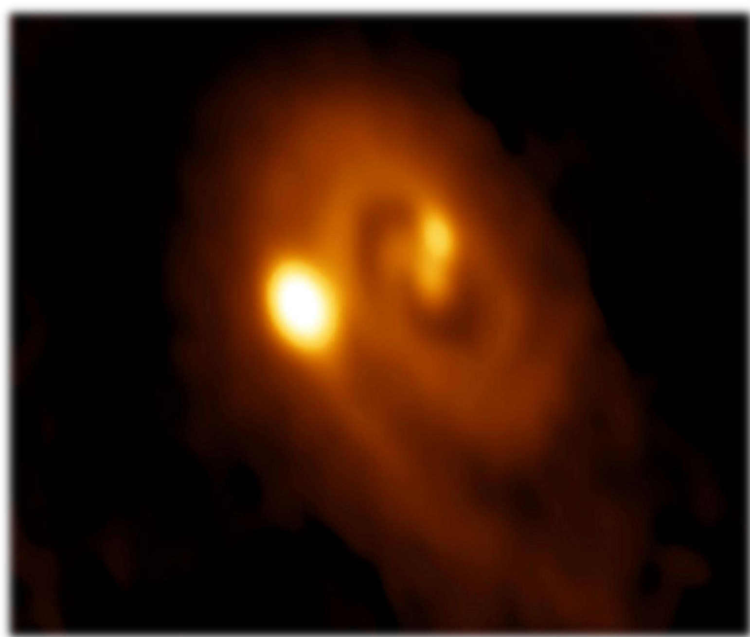
Fig. 1. De mechanismen van stervorming verklaren waarom een meerderheid van de sterren behoort tot een dubbele of een meervoudige ster. Les mécanismes de formation stellaire permettent de comprendre pourquoi la majorité des étoiles appartiennent à des systèmes doubles et multiples. © ALMA (ESO/NAOJ/NRAO), NRAO/AUI/NSF
