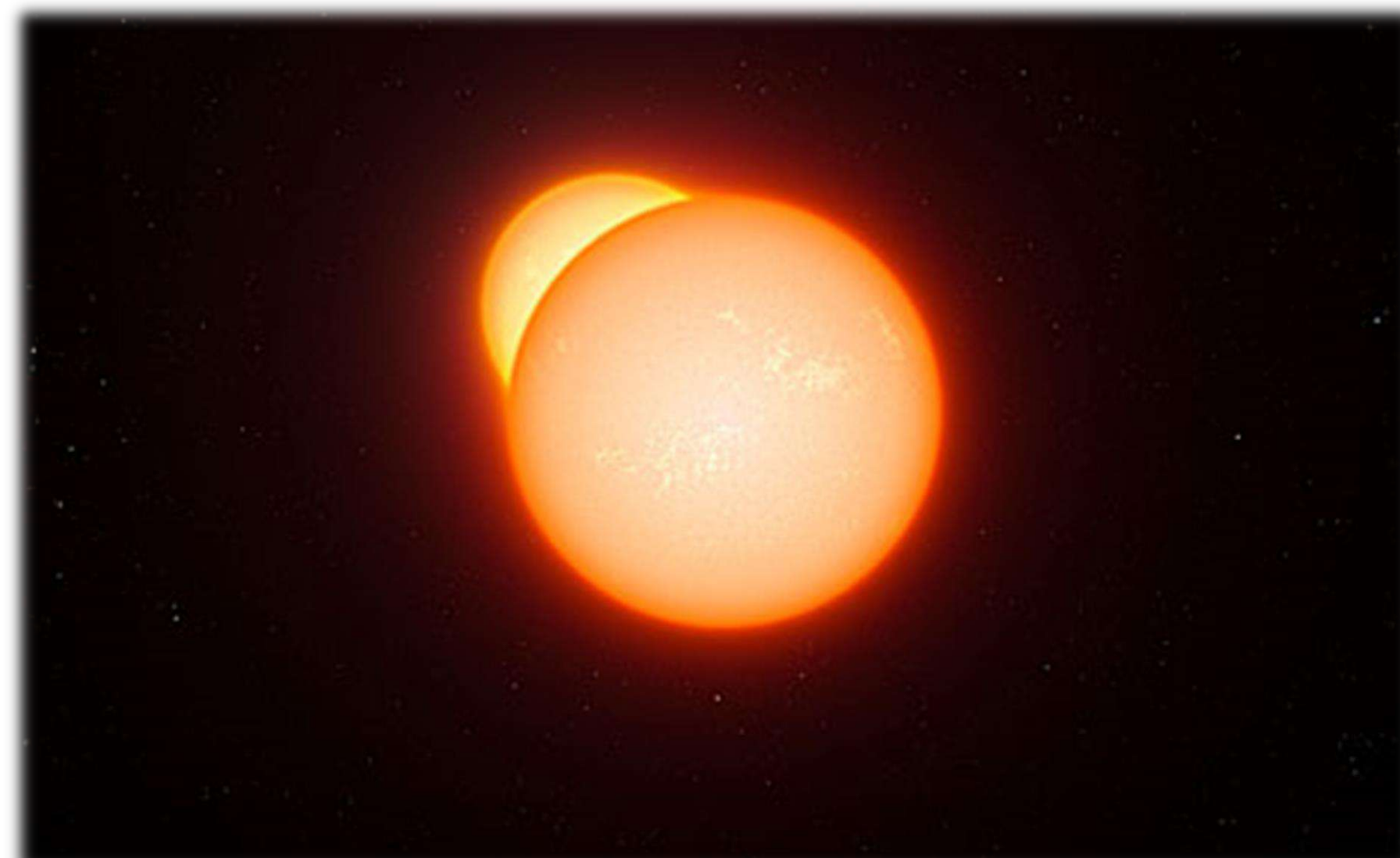
Fig. 3. Meer dan 67% van de sterren uit de nabije zonsomgeving behoren tot dubbele of meervoudige stersystemen. De zon heeft geen begeleider, wat haar vanuit dit standpunt uitzonderlijk maakt. Plus de 67% des étoiles de l'environnement solaire appartiennent à des systèmes d'étoiles doubles et multiples. Le Soleil n'a pas d'étoile-compagnon, ce qui la rend exceptionnelle vue sous cet angle. © NASA/JPL-Caltech
