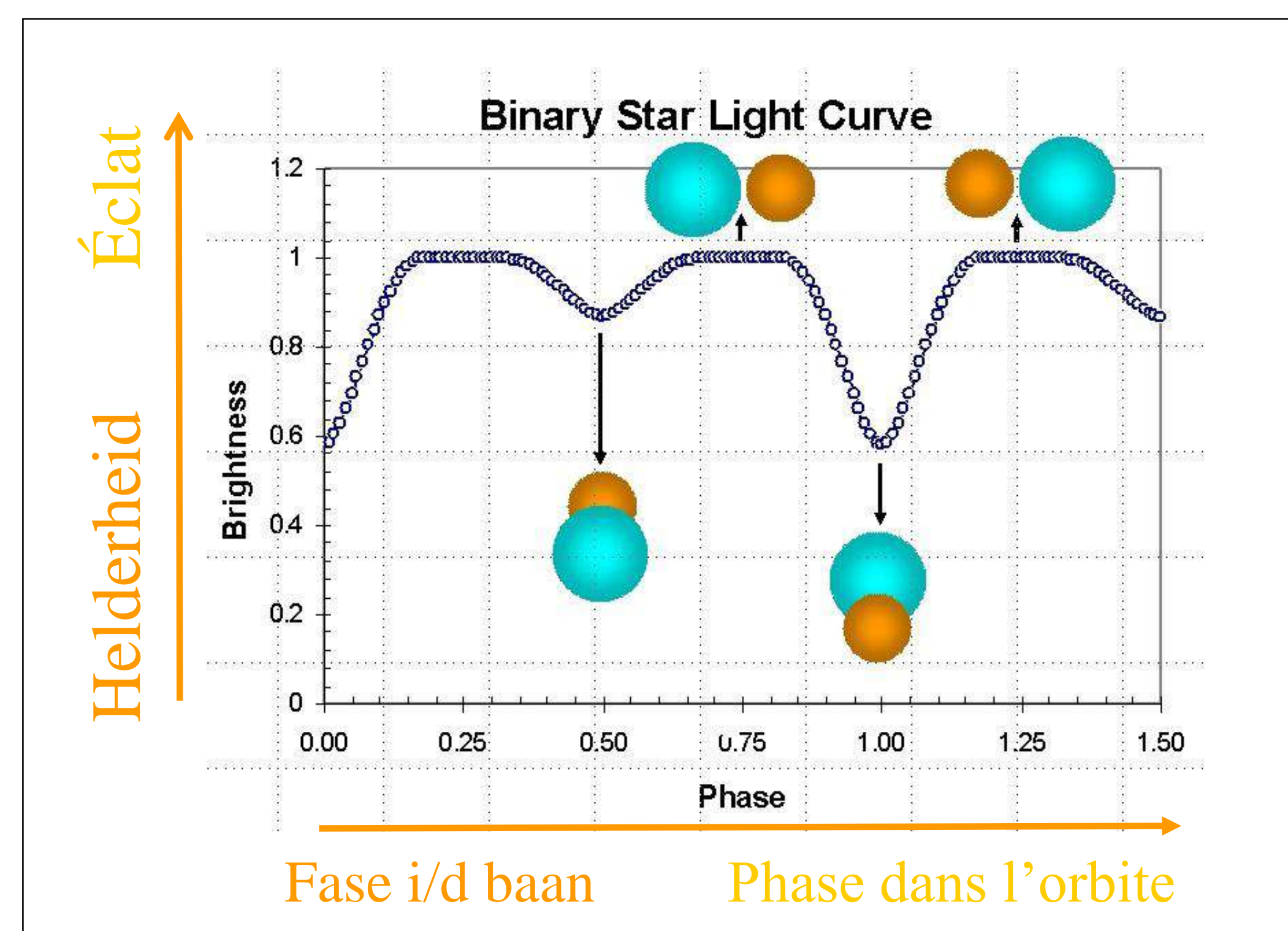
Fig. 5. De studie van de baan van een dubbelster kan, samen met de afstand tot het systeem, leiden tot de kennis van de massa van beide sterren. Daarom zijn dubbelsterren van fundamenteel belang voor de astrofysica. De periode van de baan leidt men (soms) af uit een "lichtkurve" (= verloop van de intensiteit in functie van de fase in de baan ). L'étude de l'orbite d'une étoile double permet de déterminer la masse des composantes, à condition de connaître la distance du système. C'est la raison de leur importance pour l'astrofysique. La période peut être obtenue (dans certains cas) à partir d'une "courbe de lumière" (= évolution de l'éclat total en fonction de la phase dans l'orbite).
