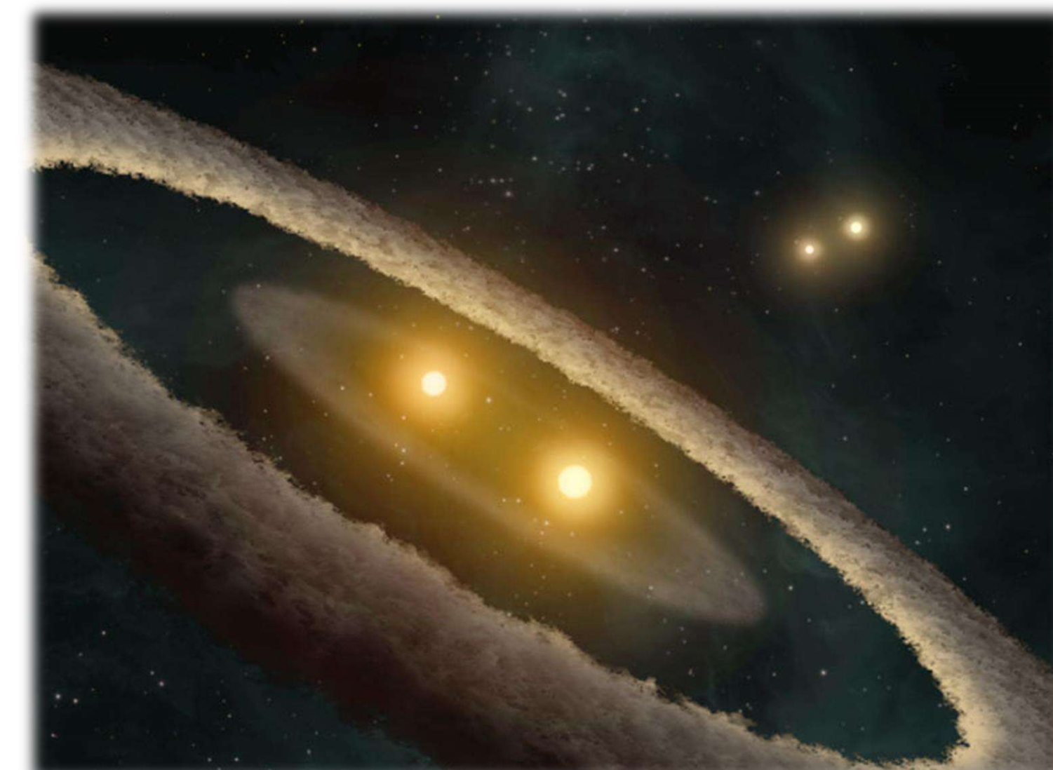
Fig. 3. Meer dan 67% van de sterren uit de nabije zonsomgeving behoren tot dubbele of meervoudige stersystemen. De zon heeft geen begeleider, wat haar vanuit dit standpunt uitzonderlijk maakt. Plus de 67% des étoiles de l'environnement solaire appartiennent à des systèmes d'étoiles doubles et multiples. Le Soleil n'a pas d'étoile-compagnon, ce qui la rend exceptionnelle vue sous cet angle. © NASA/JPL-Caltech
